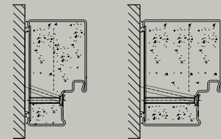
Blockzarge Typ 4.1 und Blockzarge Typ 4.2
